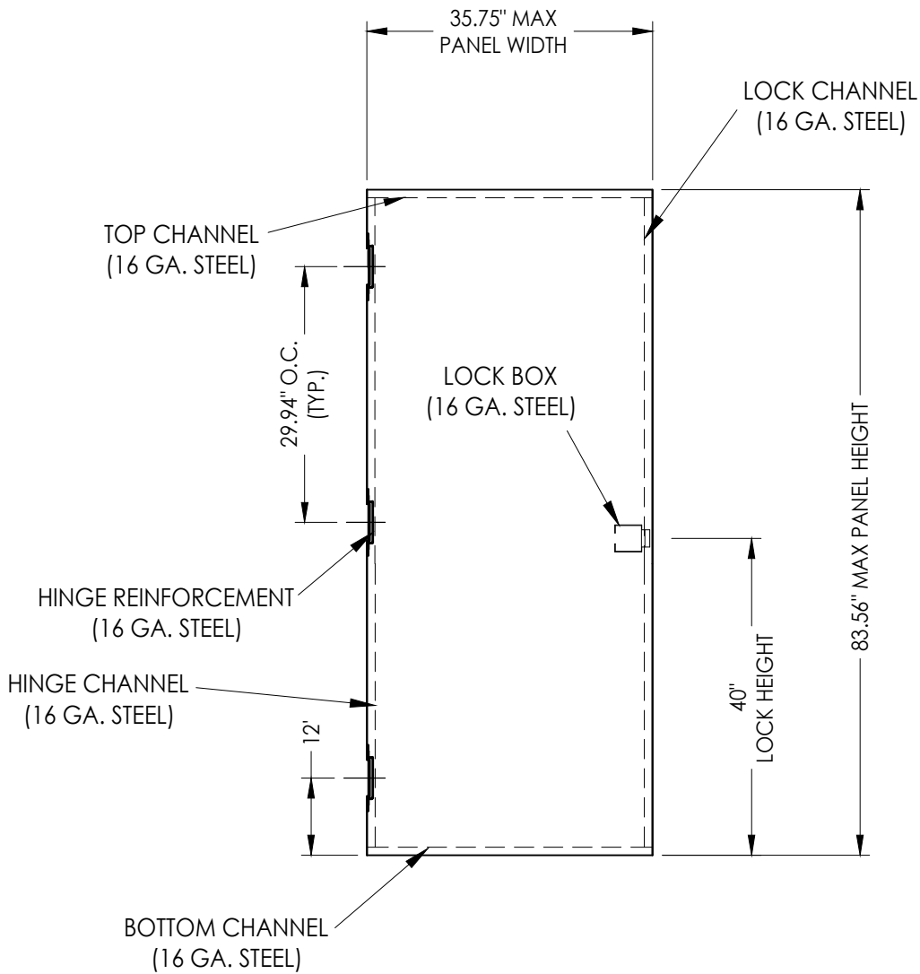
18 GAUGE STEEL DOOR PANEL STEEL DOOR SKIN: 0.044" MIN. THK.
